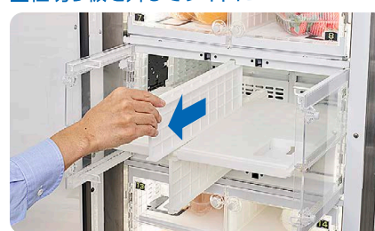
■仕切り板を外してワイドに
